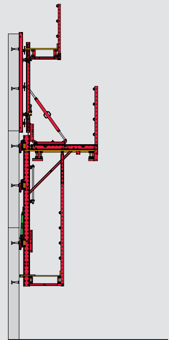
Betonowanie kolejnego etapu za pomocą lekkiego deskowania przestawnego RCS CL.
