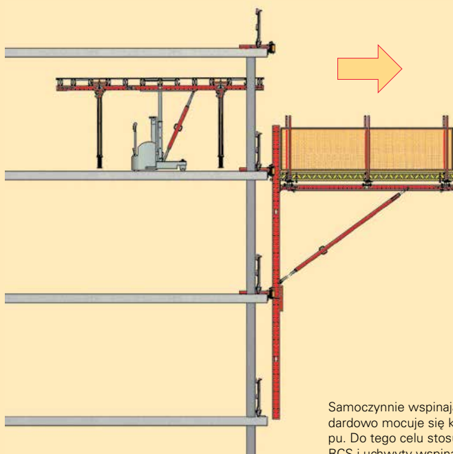
Samoczynnie wspinająca się wysuwnica RCS z dwoma podestami dolnymi jest zakotwiona w słupach obwodowych za pomocą uchwytu ściennego RCS.
