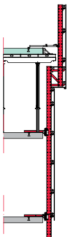
Wariant 1 Standardowy, z wąskim podestem roboczym.
