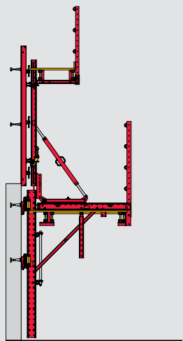
Zastosowanie RCS CL w 1. etapie betonowania.
