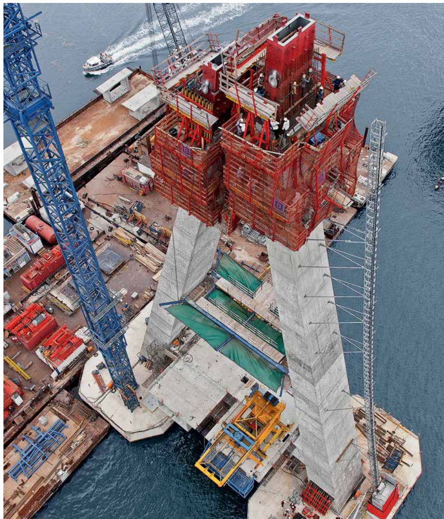
Na potrzeby realizacji pylonu mostu w Nigerii firma PERI połączyła systemy ACS i RCS. Prace wykonywane bez użycia żurawia zapewniały szybki postęp robót pomimo zmieniającego się nachylenia pylonów.
