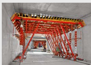
Deskowania tunelowe
