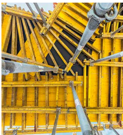
MULTIFLEX z użyciem podwójnych dźwigarów GT 24 dla optymalnego dopasowania do geometrii okrągłego zbiornika.
